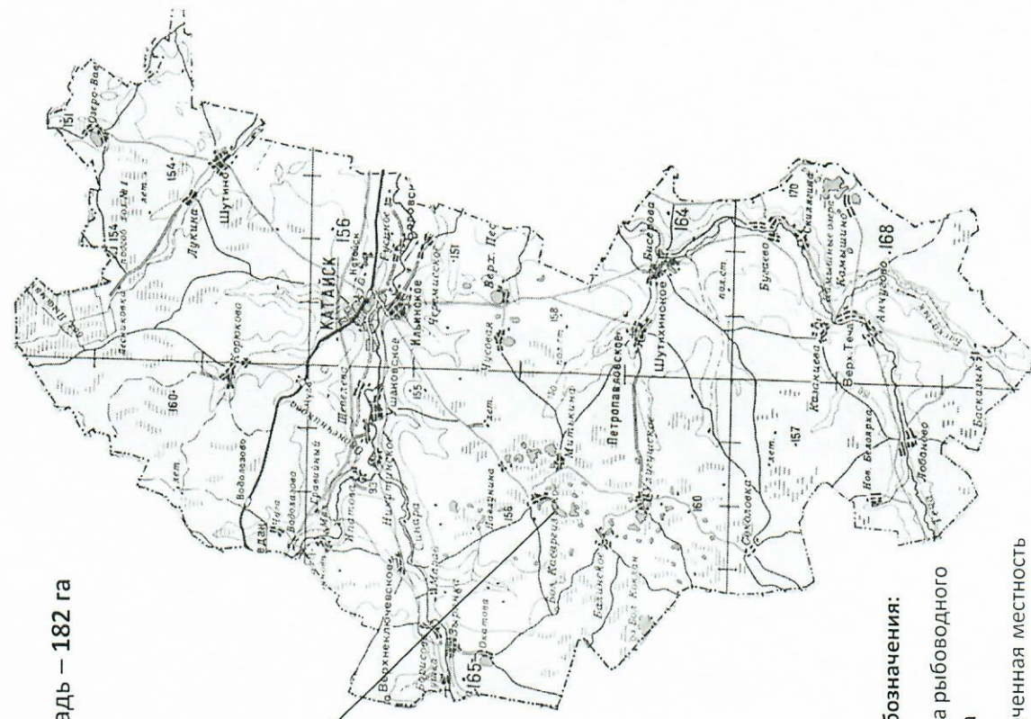
оз. Касаргуль
